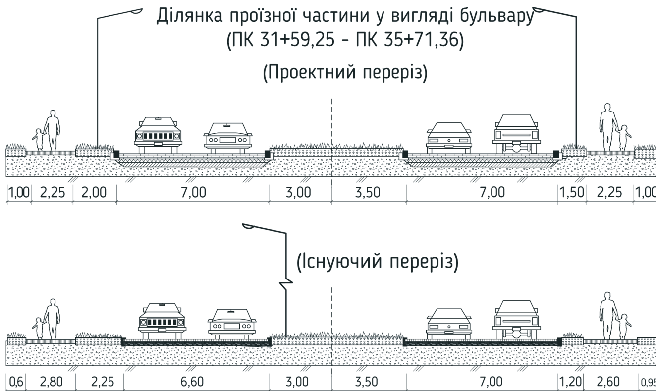
Рисунок – Поперечний профіль проектного та існуючого положення проїзної частини у вигляді бульвару.
