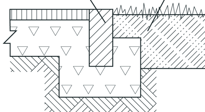
Рисунок – Конструкція дорожнього одягу на проїзній частині.
