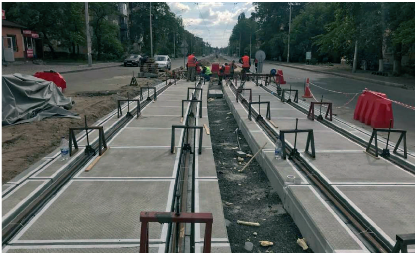
Рисунок – Рейки 60R2 вивішують і виставляють на проектні вертикальні відмітки
