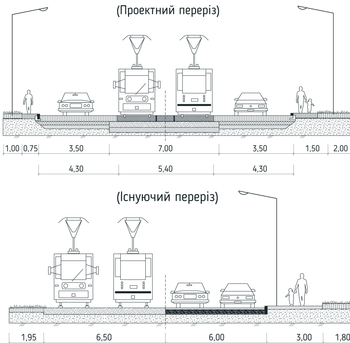
Рисунок – Поперечний профіль проектного та існуючого положення трамвайних колій на рівні з проїзною частиною від вул. Трактористів до вул. О. Довбуша.
