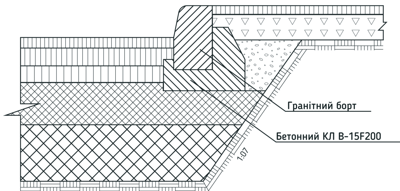
Рисунок – Конструкція дорожнього одягу на проїзній частині.
