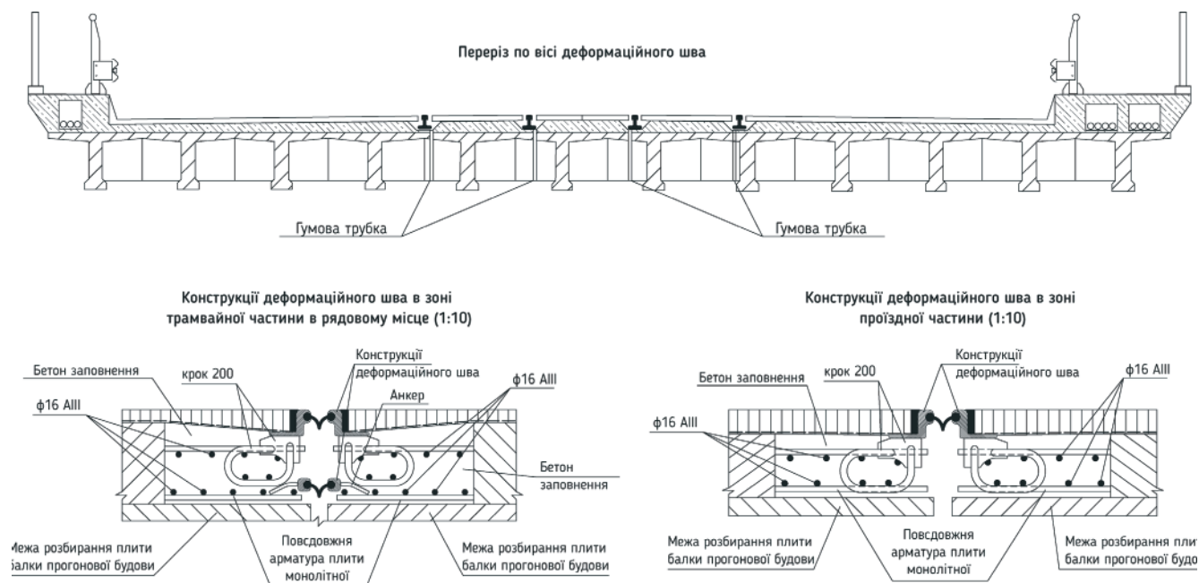
Рисунок – Проектне рішення по конструкції деформаційного шва в зоні проїздної частини мостового полотна
