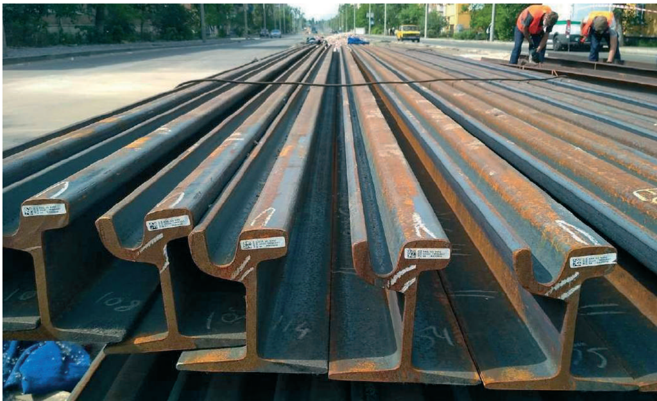
Рисунок – Трамвайні рейки 60R2
