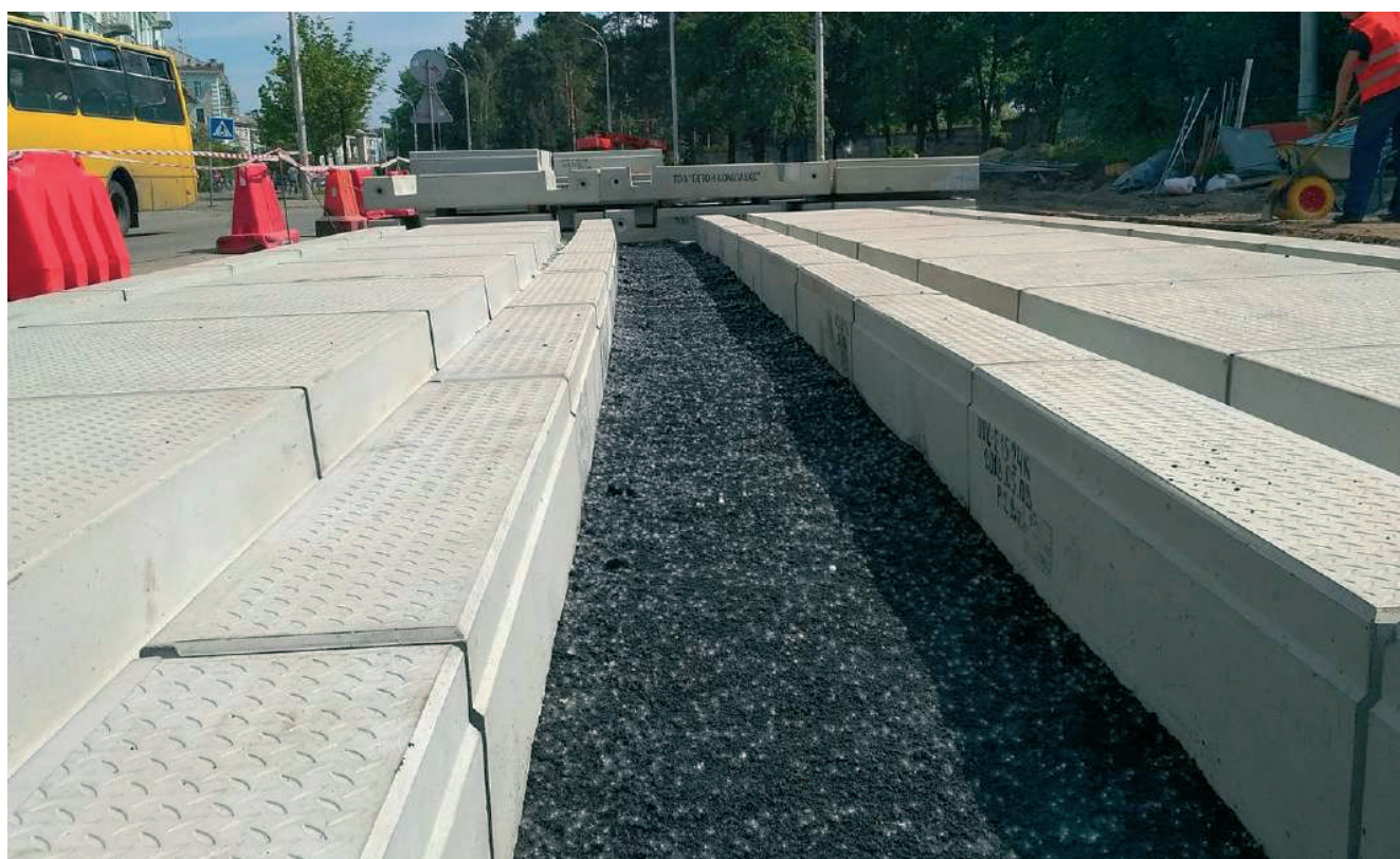
Рисунок – Після укладання георешітки і поетапного засипання та ущільнення щебеню товщиною 120 мм фракцією 40-70 та 80 мм фракцією 20-40 мм, поверхню щебеневу подушку проливають бітумною емульсією (витрата 2,5 л/м 2 ) для кращого зчеплення дрібнозернистого асфальтобетону фракцією 10 мм (шар 3 см), який виконує функцію вирівнюючого шару та є підосновою. Влаштування бетонного шару товщиною 200 мм
