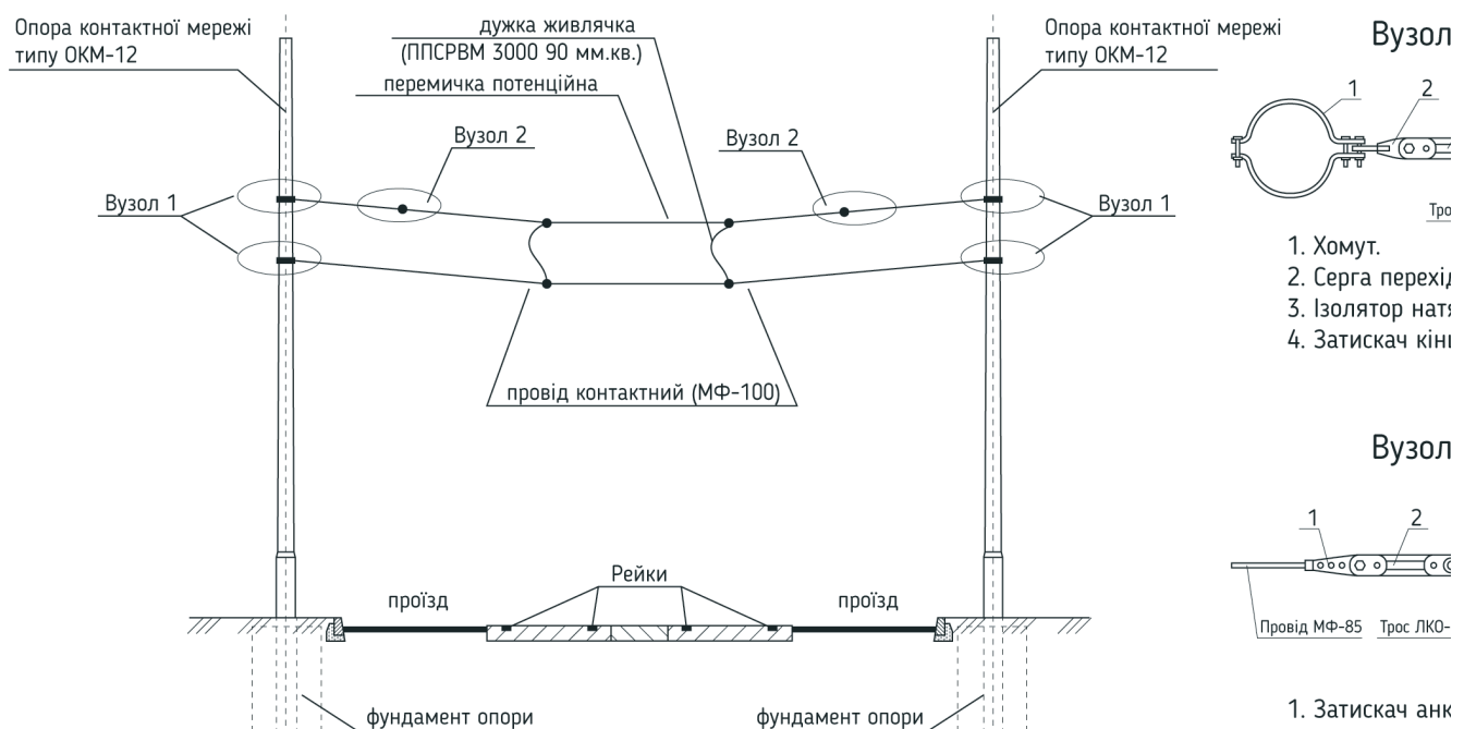
Рисунок – Проектна схема контактної підвіски потенційна перемичка (+600 В)
