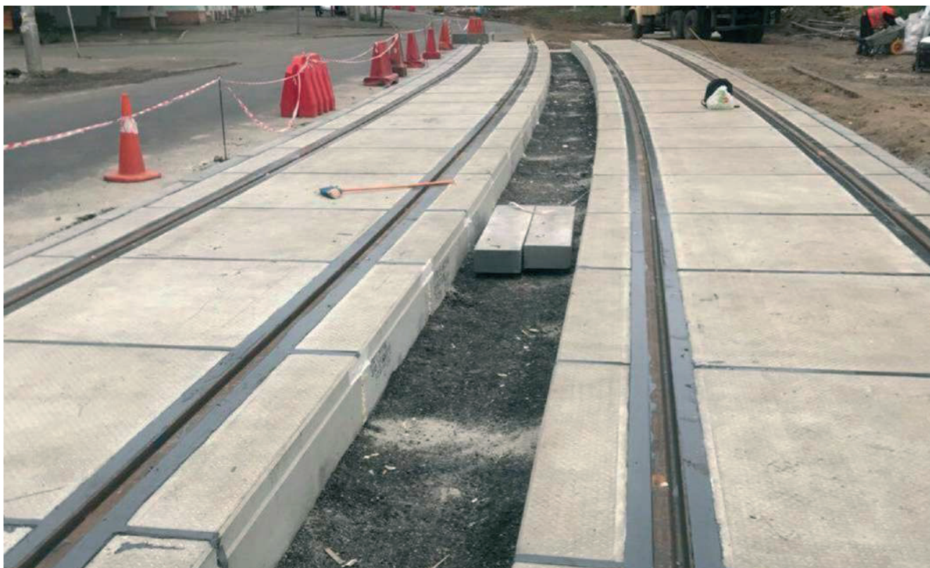
Рисунок – Рейки 60R2 заливають поліуретановим матеріалом Sika Icosit KC
